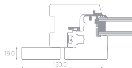
Nodo laterale finestra e porta finestra
