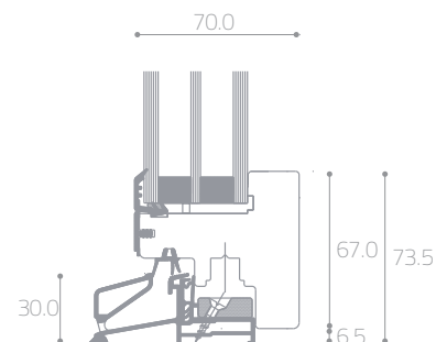
Nodo inferiore porta finestra
