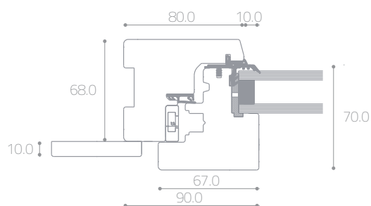
Nodo in pianta della finestra e della porta finestra
