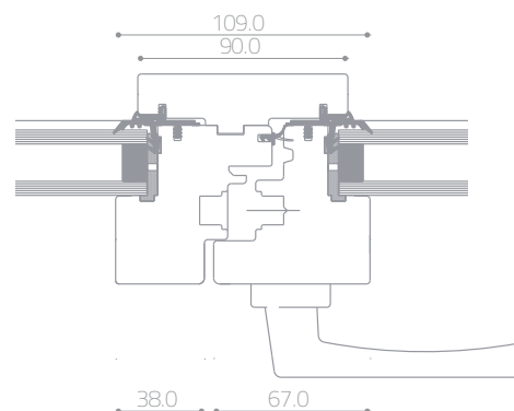
Nodo centrale asimmetrico
