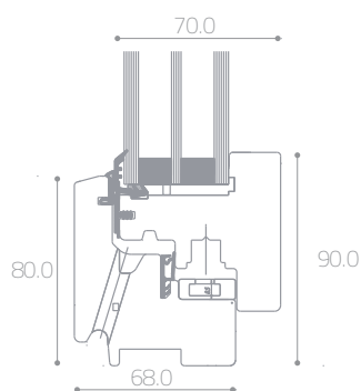
Nodo inferiore finestra
