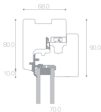
Nodo superiore finestra / porta finestra
